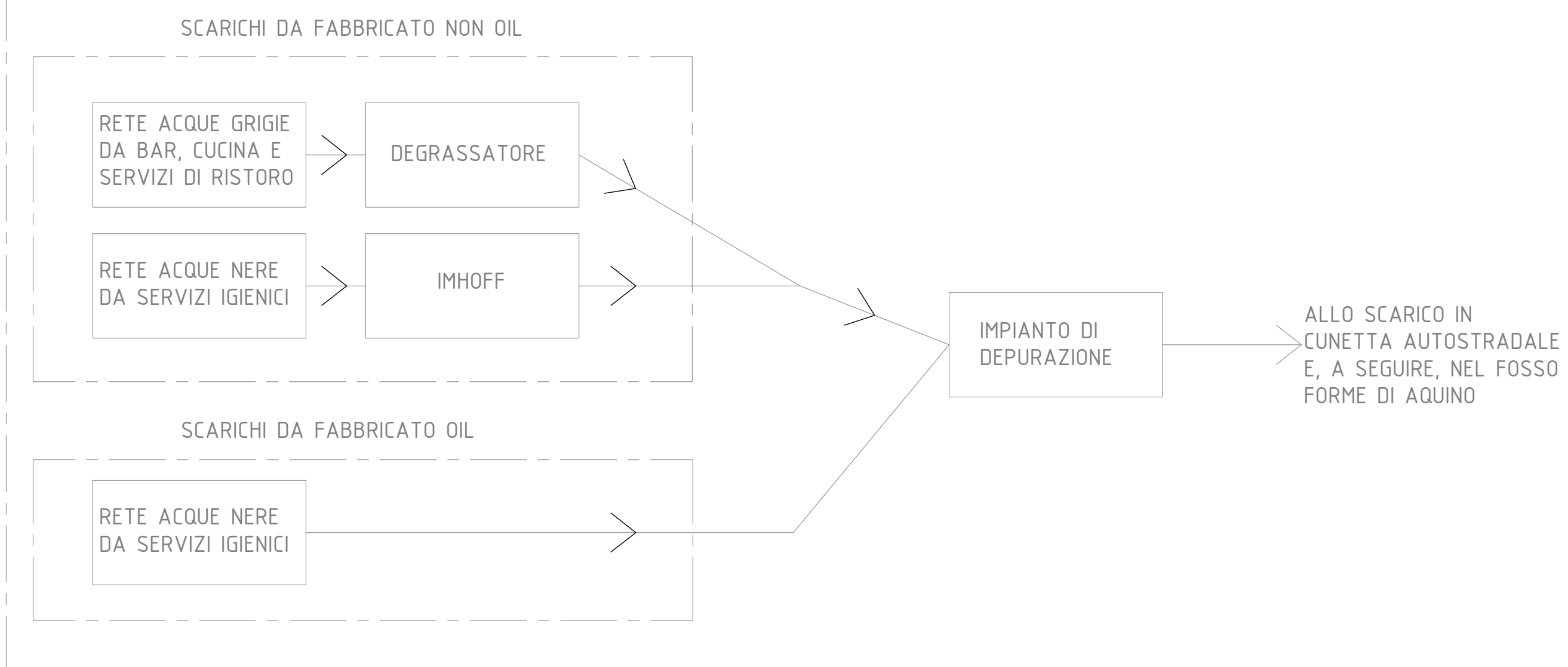
SCHEMA A BLOCCHI ACQUE REFLUE ASSIMILATE ALLE DOMESTICHE
