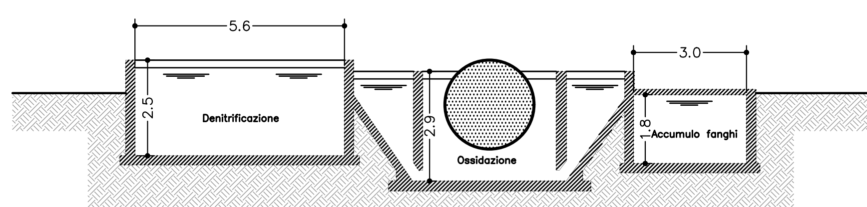
Sezione A-A - scala 1:100
