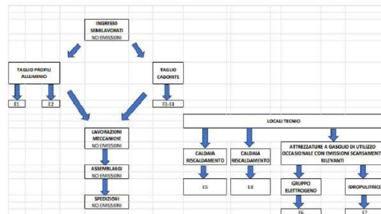
DIAGRAMMA A BLOCCHI CICLO PRODUTTIVO
