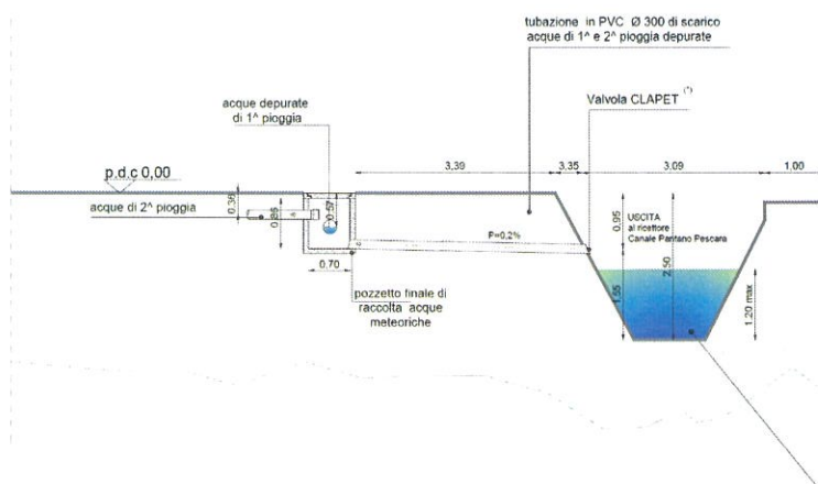
PARTICOLARE SCARICO ACQUE DI 1^ e 2^ PIOGGIA
